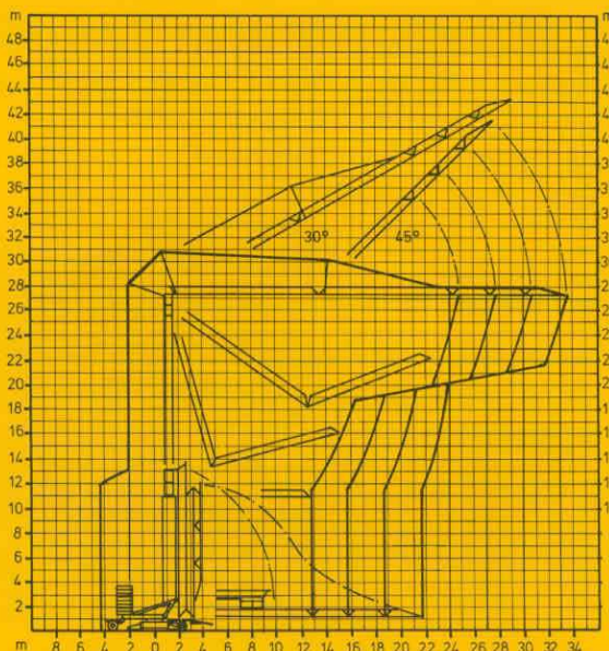
Ballasterausladung 5,0 m Ballasting radius 5,0 m Portée pour dispositif de lestage 5,0 m
